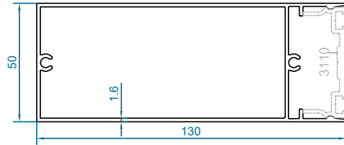
code : 3111 پروفیل درپوش 130 Box Cover Profile weight :1.69kg/m
