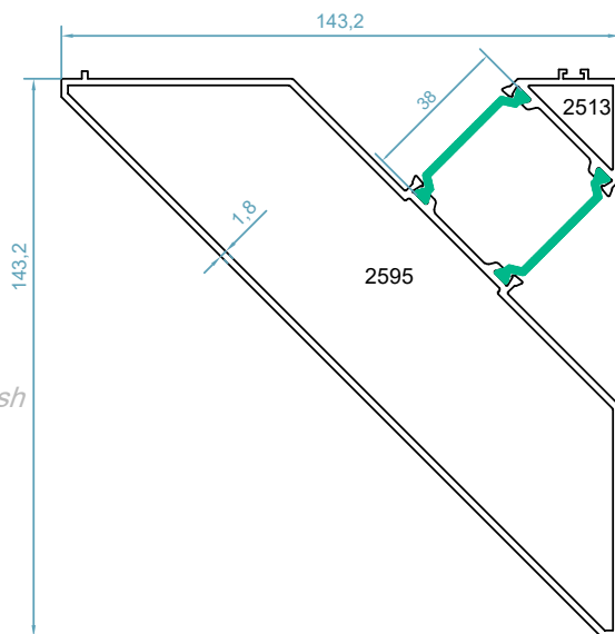
code : 2513-2595 آداپتور کنج فریم دو ریل corner adapter weight: 3.18kg/m
