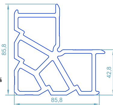
code : 112 گونیا پانچی Corner Cleat weight : 5.00 kg/m
