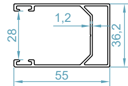
ريل آكا Aka Rail Profile code: 9155
