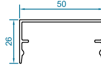
code : 3115 پروفیل درپوش Cover Cap Profile weight :0.46kg/m
