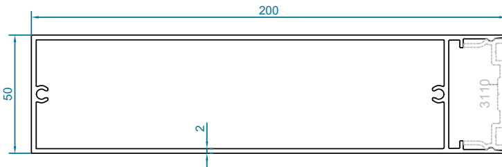
code : 3160 پروفیل درپوش 200 Box Cover Profile weight :2.97kg/m
