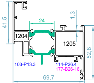
code : 1204-1205 پنجره داخل بازشو Inward Opening Window weight : 1.46 kg/m
