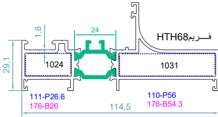
code : 1024-1031 فریم کتیبه سری TH68 hinge adjoining frame weight : 1.90 kg/m
