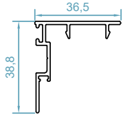
code : 2116 پروفیل اینترلاک Interlock Profile weight :0.4 kg/m
