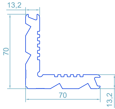
code : 111 گونیا پانچی Corner Cleat weight : 4.03kg/m
