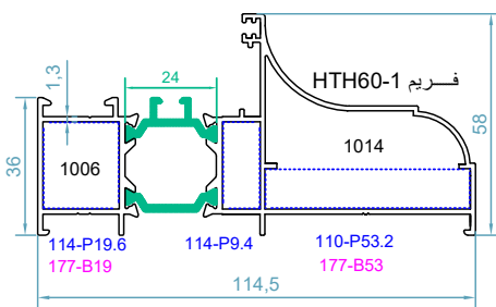
code : 1006-1014 فریم کتیبه سری TH60 hinge adjoining frame weight : 1.79 kg/m
