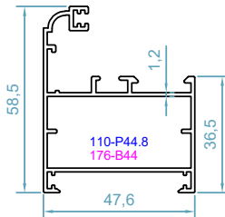
code : 1507 فریم پنجره Frame Profile weight : 0.87 kg/m Jx=9.7 \text{ cm}^4 Jy=8.9 \text{ cm}^4
