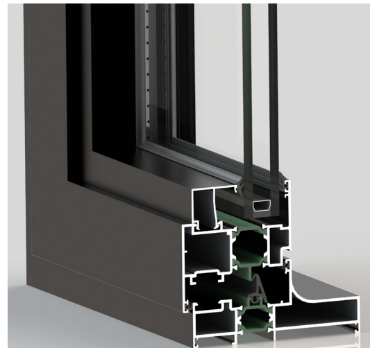
code 2014 مابین فریم و کتیبه between two frame weight : 0.14 kg/m
