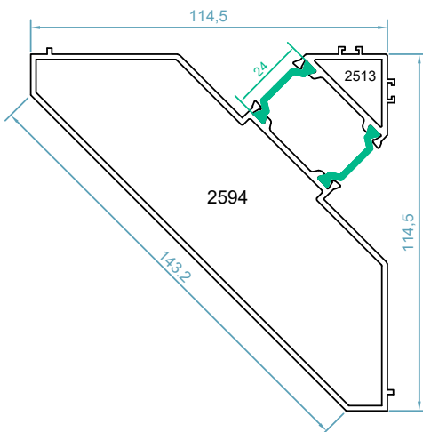
code : 2513-2594 آداپتور کنج فریم corner adapter weight : 2.7kg/m
