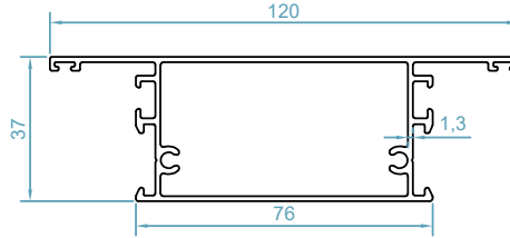
code : 1592 پروفیل سپری T Profile weight : 1.41 kg/m Jx=9.49 \text{ cm}^4 Jy=49.79 \text{ cm}^4
