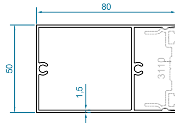
code : 3112 پروفیل درپوش 80 Box Cover Profile weight :1.26kg/m
