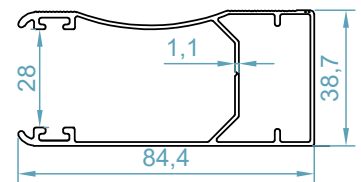
ريل الگانس Elegance Rail Profile code: 9152
