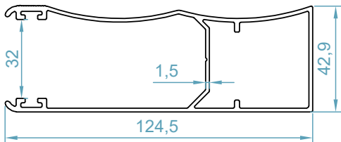
ريل نوبل Noble Rail Profile code: 9150
