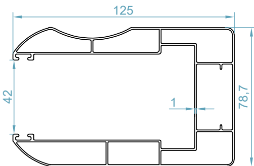
ريل جاينت Giant Rail Profile code: 9156
