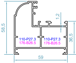
code : 1513 پروفیل فریم Frame Profile weight : 1.05 kg/m Jx=12.6 \text{ cm}^4 Jy=9.9 \text{ cm}^4
