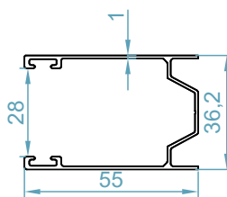
ريل بكا Beka Rail Profile code: 9157
