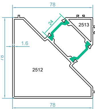
code : 2512-2513 آداپتور کنج فریم 1552 1552 Corner Adapter weight : 2.25 kg/m Jx=58.7 \text{ cm}^4 Jy=51.8 \text{ cm}^4
