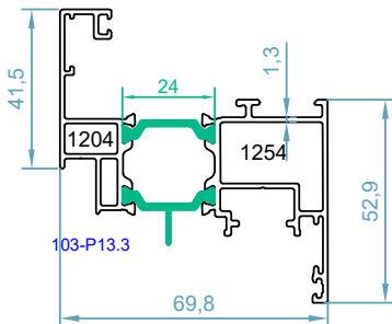
code : 1204-1254 پنجره یراق پی وی سی Sash Profile -Multi Point weight : 1.50 kg/m
