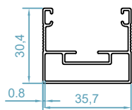
code : 2549 فریم توری پلیسه Fly Screen Frame weight : 0.34 kg/m
