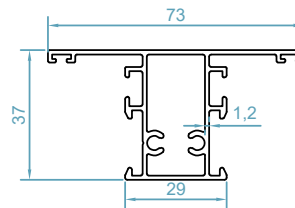
code : 1587 پروفیل سپری T Profile weight : 0.85 kg/m Jx=8.48 \text{ cm}^4 Jy=5.78 \text{ cm}^4
