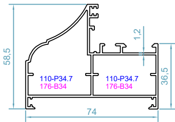
code : 1552 پروفیل فریم Frame Profile weight : 1.20kg/m Jx=18.71 \text{ cm}^4 Jy=10.95 \text{ cm}^4
