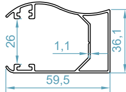
ريل نايس Nice Rail Profile code: 9154
