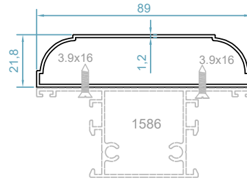
code : 2590 آداپتور سپردنصب توری Fly Screen Adapter For T Pr weight : 0.7 kg/m
