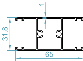
code : 2100 پروفیل سپری T Profile weight : 0.651 kg/m
