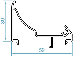
code : 2518 آداپتور گردان فریم 1513 1513 Corner Adapter weight : 0.57 kg/m
