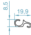
پروفیل غضروف Lux M 70 Shutter برای لوکس 70 code: 9022
