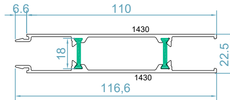
code :1430-1430 ورق دو جداره ی ترمال بریک Thermal Break Shutter Pr. weight : 1.5 kg/m
