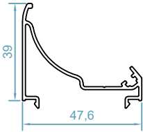
code : 1508 آداپتور گردان فریم 1507 1507 Corner Adapter weight : 0.48 kg/m
