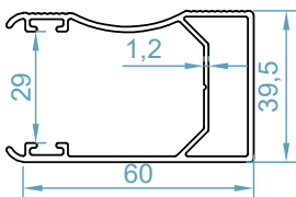
ريل ساني Sunny Rail Profile code: 9153
