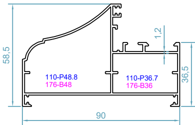
code : 1506 پروفیل فریم Frame Profile weight : 1.25 kg/m Jx=35.25 \text{ cm}^4 Jy=11.95 \text{ cm}^4
