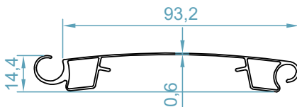
تیغه اکسترا پانچ Extra Shutter code: 9024
