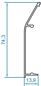
code : 3117 درپوش افقی Cover Cap Profile weight :0.39kg/m
