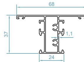
code : 1590 پروفیل سپری T Profile weight : 0.74 kg/m Jx=4.96 \text{ cm}^4 Jy=5.38 \text{ cm}^4
