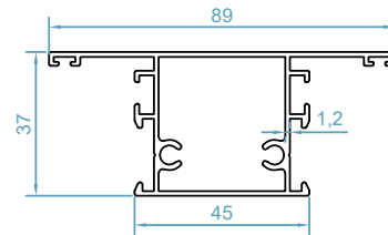
code : 1586 پروفیل سپری T Profile weight : 1.00 kg/m Jx=15.7 \text{ cm}^4 Jy=7.1 \text{ cm}^4
