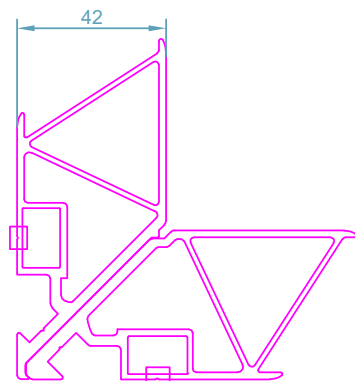
code : 179 PC B42
