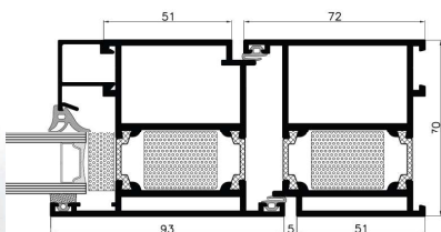
door profile MB-70 HI
